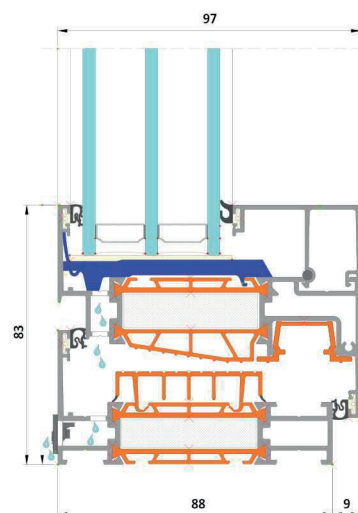
VERTIKÁLNÍ ŘEZ
