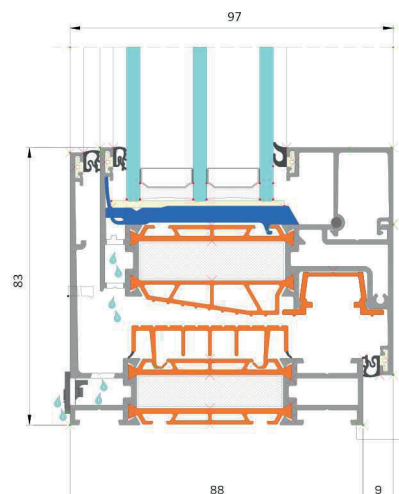
VERTIKÁLNÍ ŘEZ
