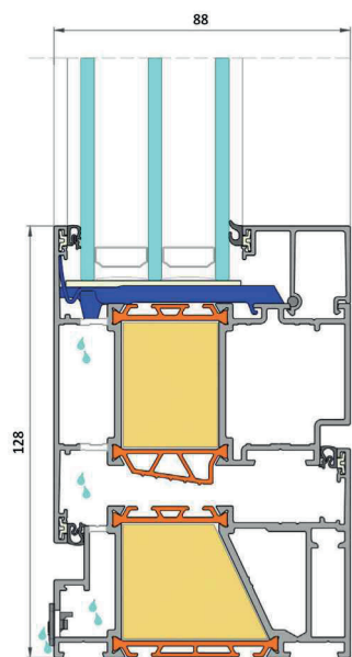
VERTIKÁLNÍ ŘEZ
