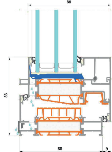
VERTIKÁLNÍ ŘEZ
