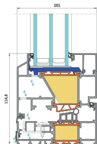
VERTIKÁLNÍ ŘEZ
