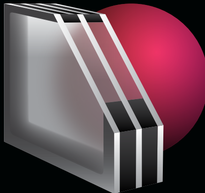
◀ Izolační trojsklo pro jednostranně překrytou hliníkovou dveřní výplň. Skladba skel dle technického popisu.
