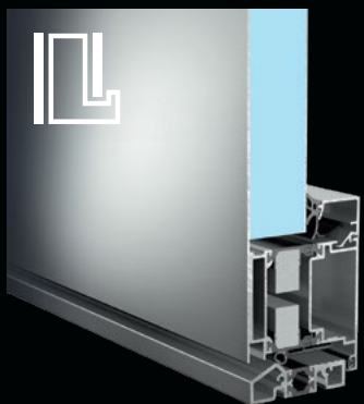
◀ Řez hliníkovým profilem s jednostranně překrytou hliníkovou dveřní výplní.
